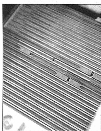
Le masque crée de minuscules fentes et cible les étoiles que les astronomes souhaitent observer. PHOTO GALLEY
