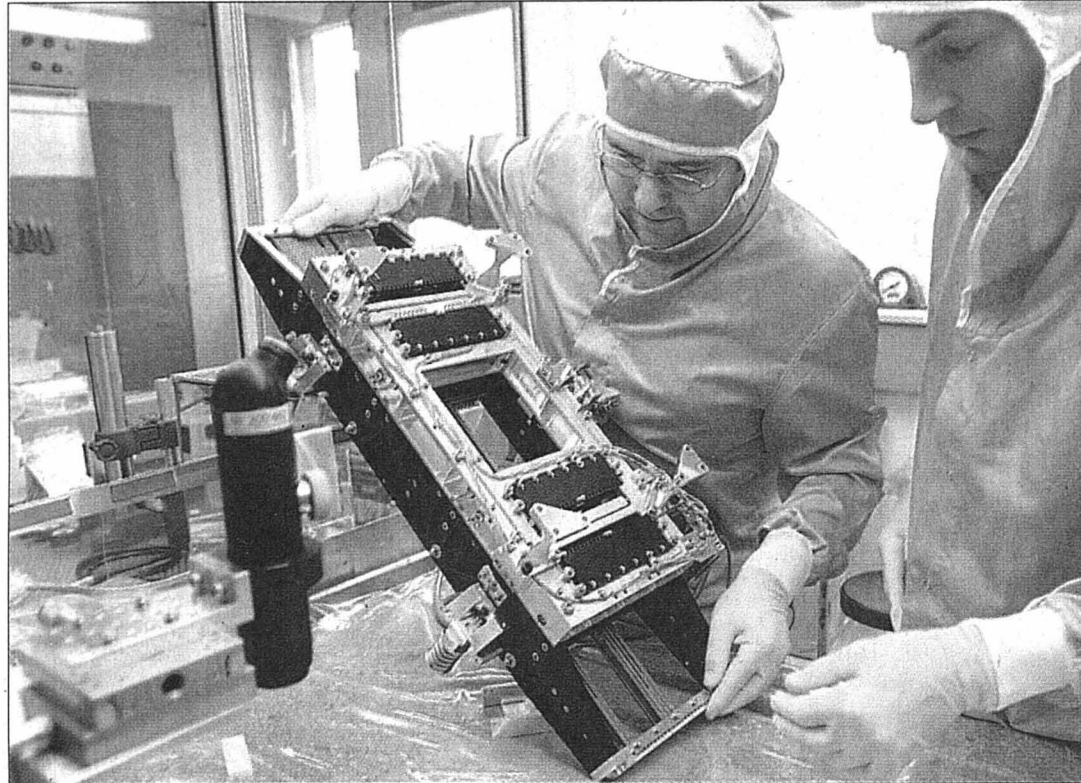
Ce masque multifentes devrait être installé sur le futur télescope spatial James Webb. PHOTO GALLEY
