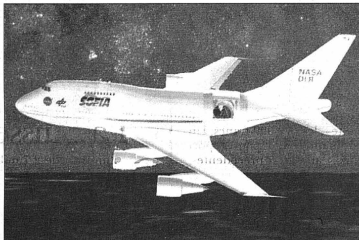
Un Boeing 747 hébergera, dès 2005, un grand télescope. DOCUMENT SOFIA
