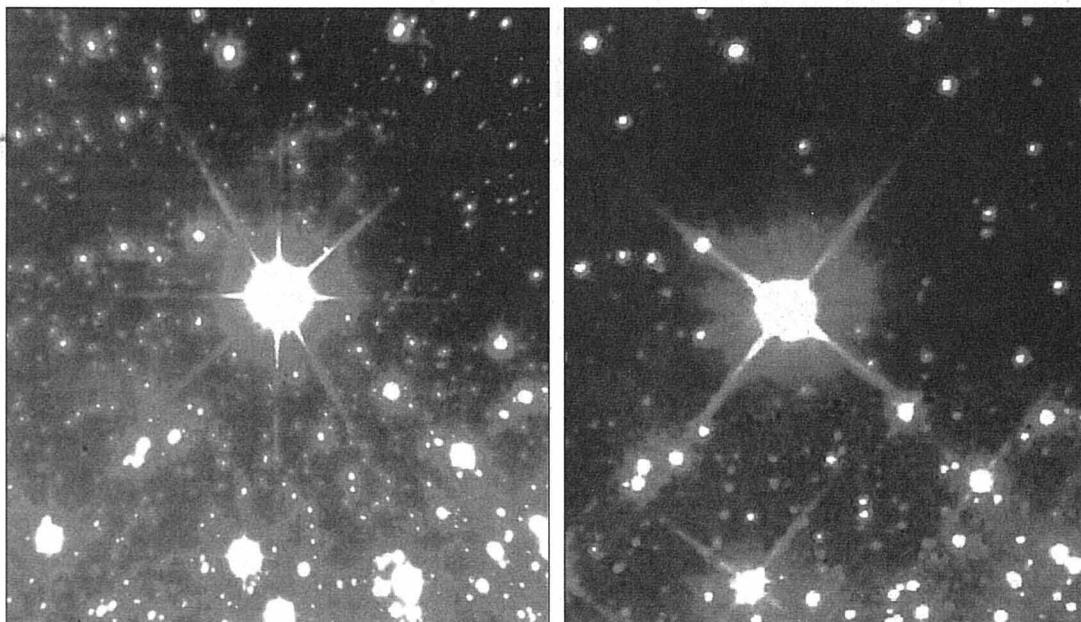
Tout est dans le détail: à droite, une image du télescope spatial Hubble. A gauche, le même ciel, mais observé à terre, au Chili, grâce à une technologie du CSEM. PHOTOS ESO
