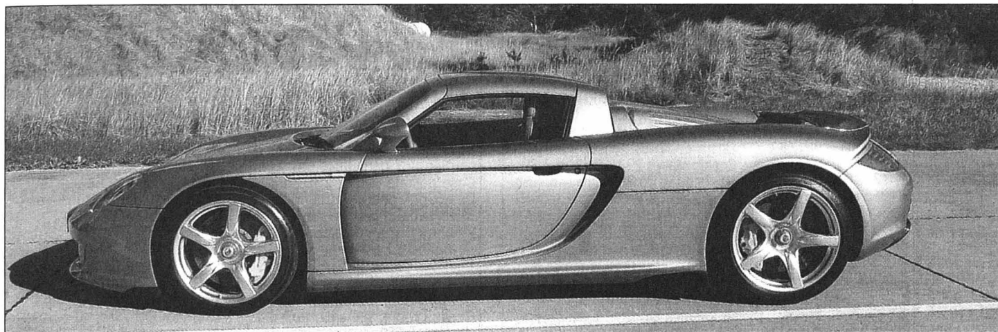
Les deux coques en carbone qui forment le toit, à 116 cm du sol, peuvent être rapidement déposées et logées dans le coffre, sans réduire sa contenance de 76 litres!
