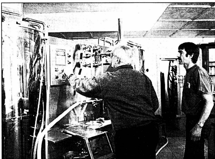
La pièce maîtresse de la microbrasserie du café du Marché, au Locle. A gauche, la cuve de brassage et, à droite, celle de filtration. Claude Gorza (aux manettes) passe la main à François Daucourt, qui pilotera le bijou, fabriqué en Italie.
