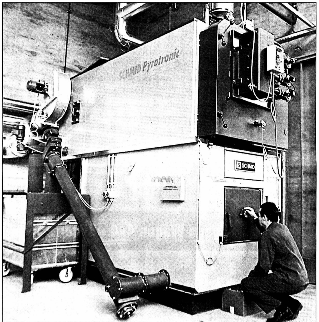
La chaudière à bois flambant neuve. PHOTO LEUENBERGER
