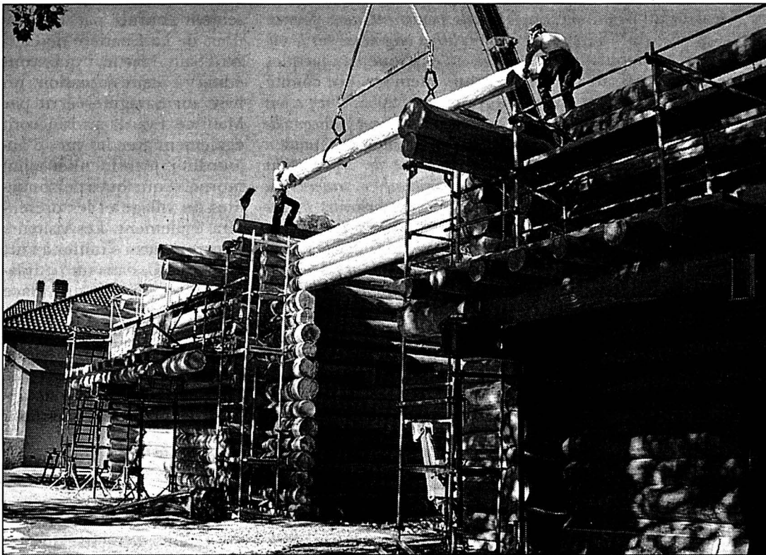
C'est le premier bâtiment du canton, de cet imposant volume, à être érigé avec des bois ronds.
