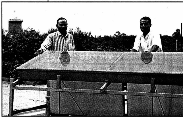
A Ouagadougou, l'atelier du CEAS a développé un capteur solaire destiné à l'alimentation d'un frigo. photo sp
