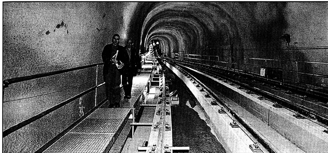
Le chemin de fuite (à gauche) consiste en un caillebotis de 80 centimètres de large. photo Marchon
