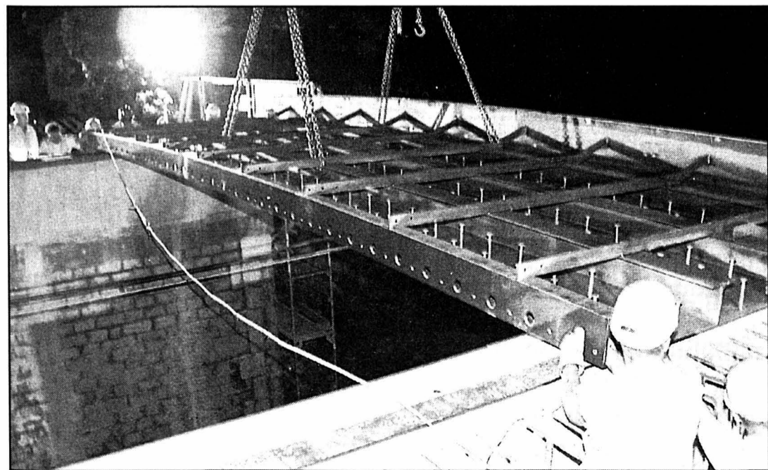
La pose des deux éléments métalliques du nouveau pont s'est faite avec une dextérité remarquable. photo Di Lenardo
