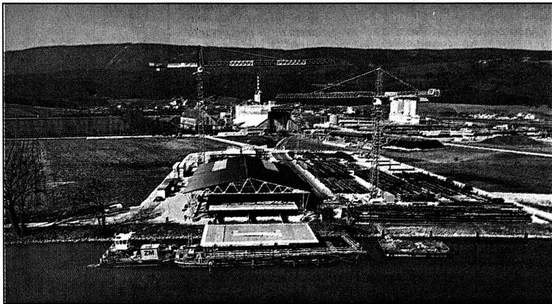
La place logistique d'Expo.02 à Cornaux. Sur la droite, les tuyaux destinés à de futurs pieux. Derrière le chaland prêt à partir avec un morceau de plate-forme, la halle de montage. photo Bettinelli
