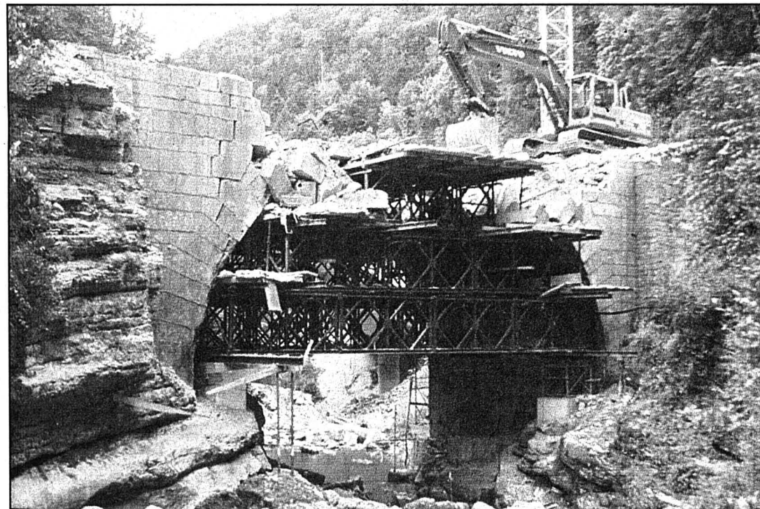
L'étaillage a évité que le pont ne s'effondre dans le Seyon. photo Galley
