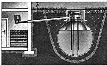
citerne enterrée
