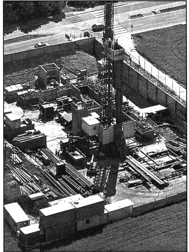
Chantier de forage (2000 m de profondeur) à Reinach, près de Bâle. photo Ofen
