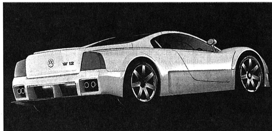
Deux VR 6 animent la Volkswagen W 12.
