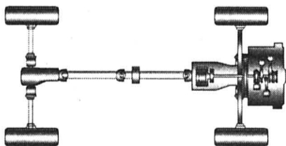
La recette de Subaru pour un comportement routier optimal: un moteur boxer qui abaisse le centre de gravité, et la traction intégrale.
