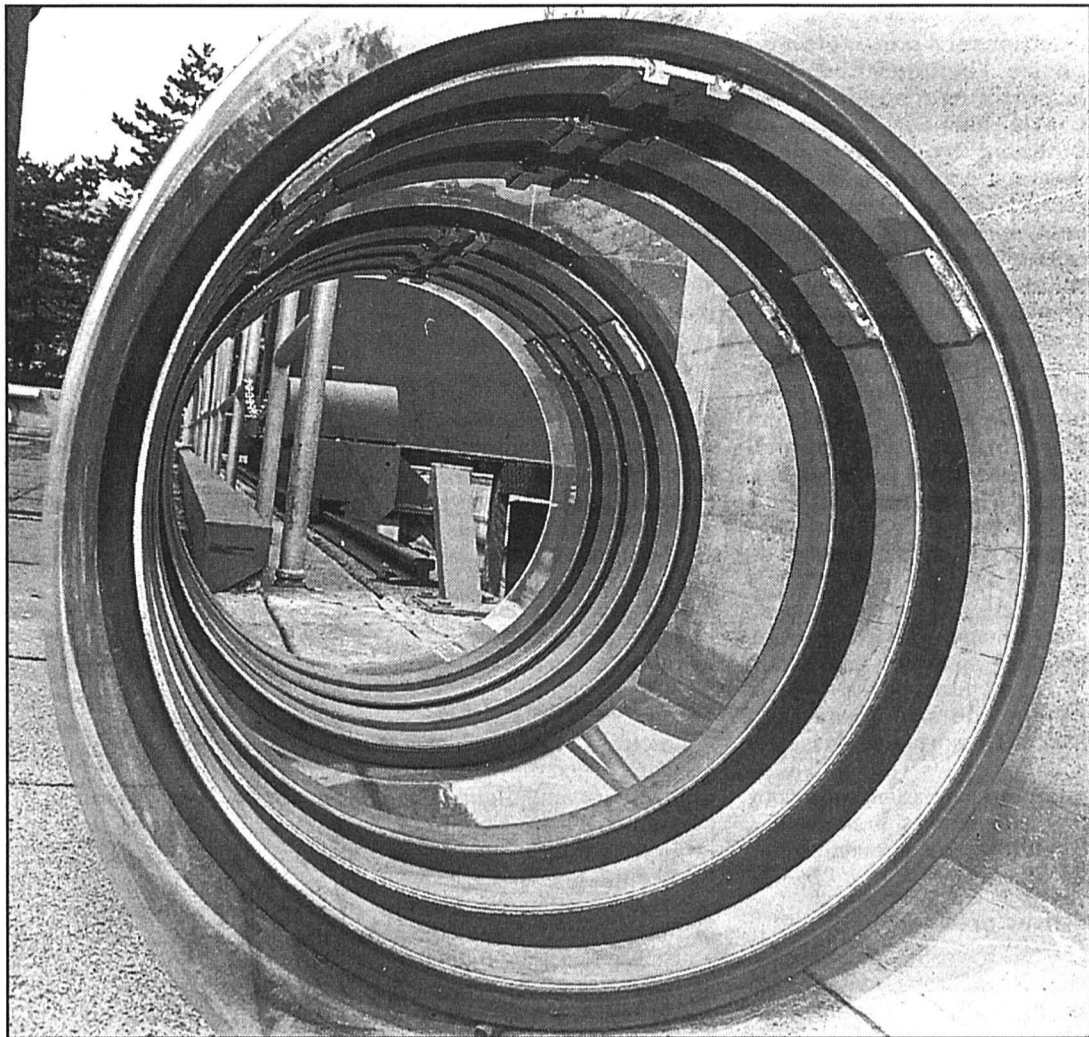
Manchons de caoutchouc souple destinés à être plaqués à l'intérieur du tuyau défectueux au moyen de cerceaux en acier inox. photo Galley
