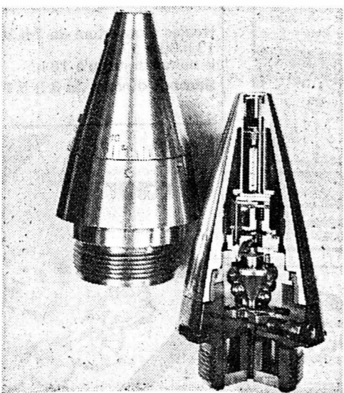
Fusées mécaniques d'artillerie avec mouvement d'horlogerie
