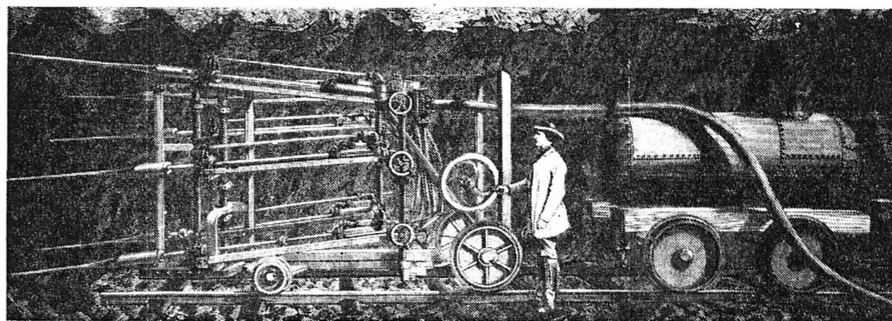
La curieuse machine à percer le tunnel du Saint-Gothard, il y a cent ans! (Keystone)
