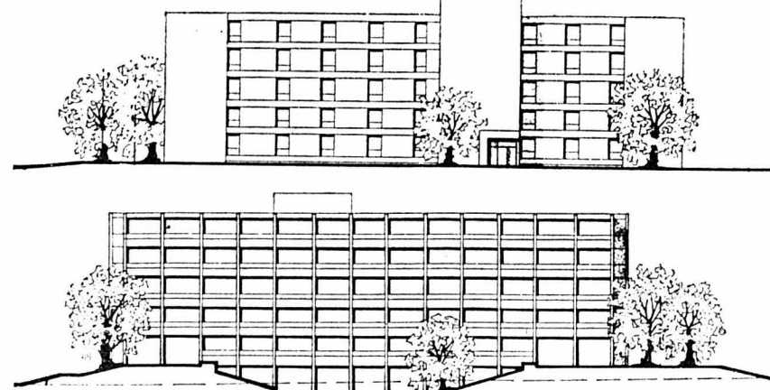
Vue des deux façades principales (nord et sud) de la future maison réservée aux personnes âgées, pour laquelle le Conseil général a voté lundi soir une subvention de 621.000 fr., en accordant à la fondation qui fera construire ce bâtiment à la Coudre, en bordure sud de la rue de la Dime, à la limite d'Hauterive, un droit de superficie de 1260 m2 pour 221.000 francs. ● Ce bâtiment comprendra 49 studios, 9 appartements de deux chambres répartis sur cinq niveaux et adaptés à leur fonction. Ce sera la troisième construction de ce genre à Neuchâtel, après celles des Cadolles et du Verger-Rond.
