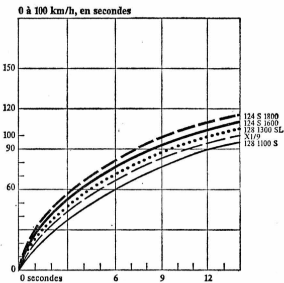
Consommation d'essence (kilomètres parcourus par litre d'essence à 100 km/h)
