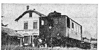
L'automotrice alors qu'elle circulait sur la ligne Uerikon-Bauma. (Photo U.S.T.)
