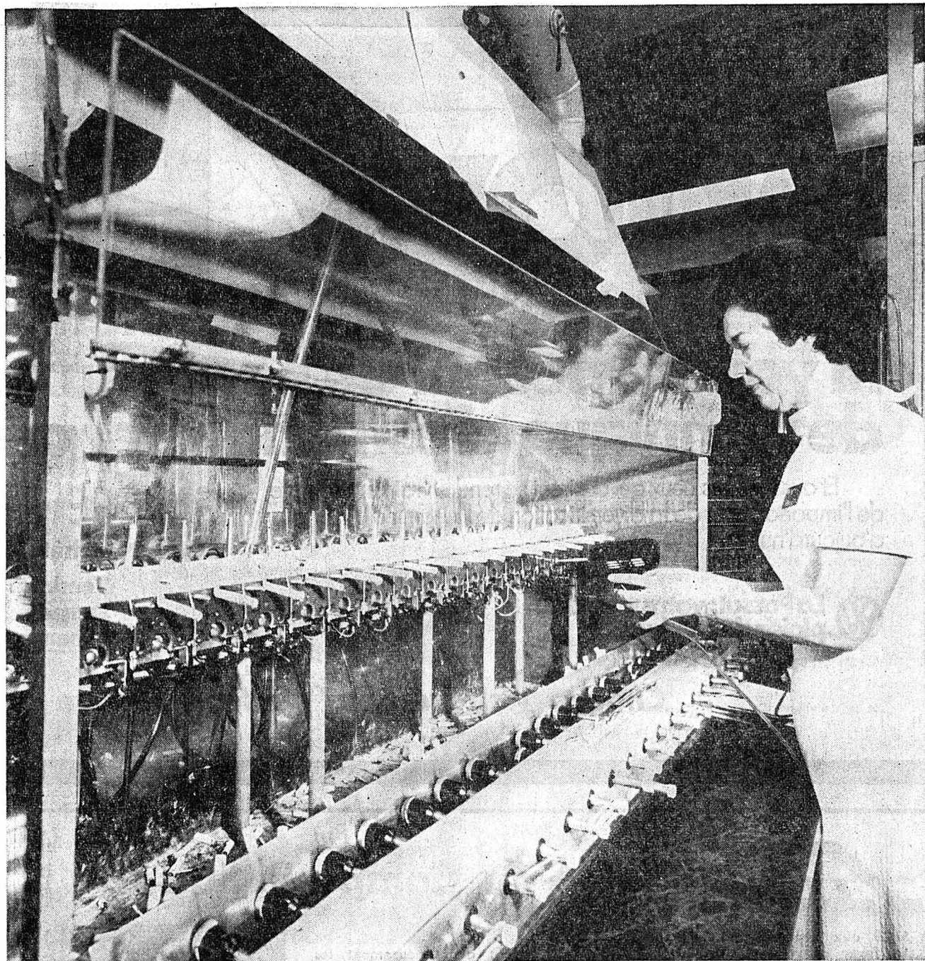
L'instrument clé dans les recherches sur le tabac : la machine à fumer, que l'on retrouve ici dans les laboratoires de Philip Morris, à Richmond (Virginie).
