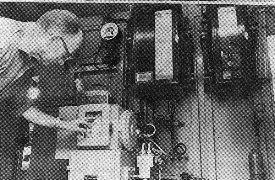
Les installations provisoires de la Maladière qui servent à injecter du gaz butane dans le gaz de ville pour alimenter tous les appareils de la région neuchâteloise qui sont déjà adaptés au gaz naturel qui sera fourni dès les premiers jours d'octobre.
