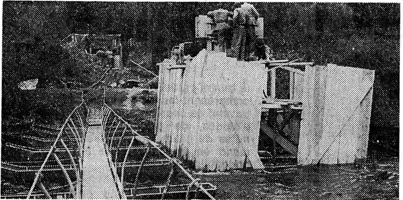
La construction de la passerelle, assurée par une troupe de génie de l'armée. (Avipress - Bévi)
