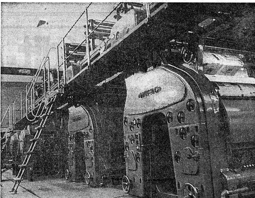
Rotative à journaux
