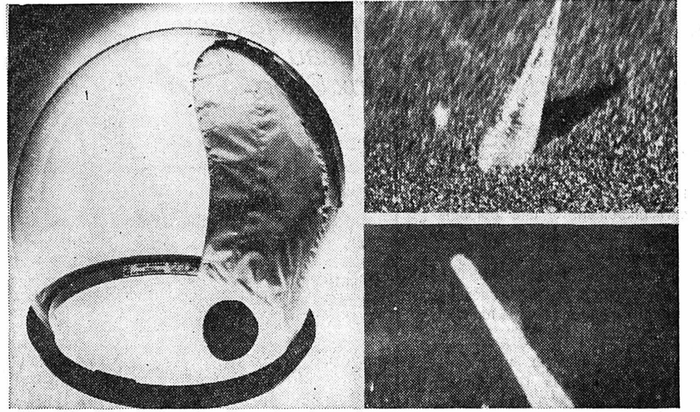
A gauche, le casque de James Lovell (Apollo-8), un de ceux qui ont servi aux études des chercheurs américains, à l'université de Berkeley notamment. A droite, les traces laissées dans l'un des casques utilisés lors d'Apollo-12.
