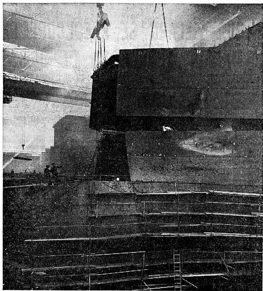
L'assemblage des tôles transportées par ponts roulants.
