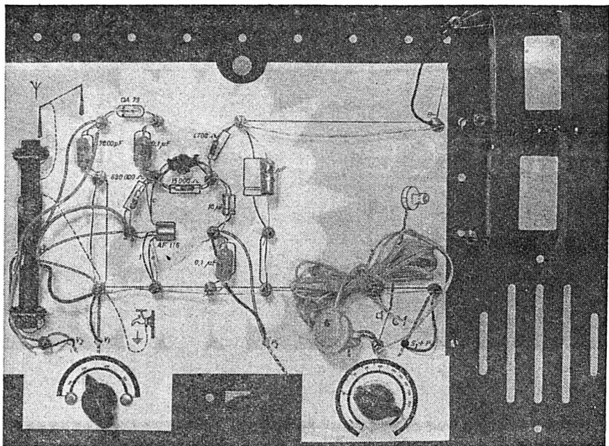
Récepteur avec un écouteur pour le futur radiotélégraphiste.
