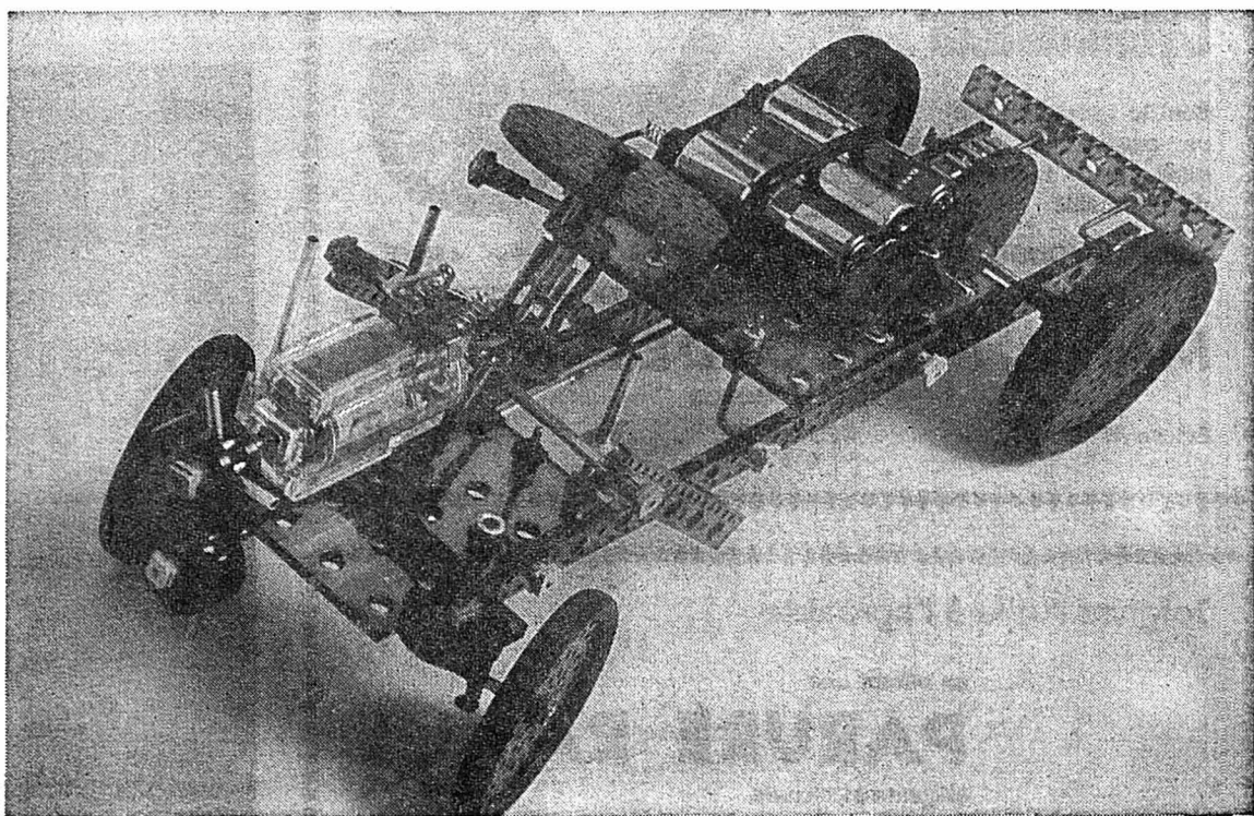
Véhicule à piles, réalisé avec une boîte de montage mécanique.
