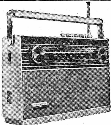
FW 509 Radio portatif, OUC/OM/OL/OC, réglage de tonalité, 249 x 164 x 67 mm, 1,5 kg Fr. 175.—
