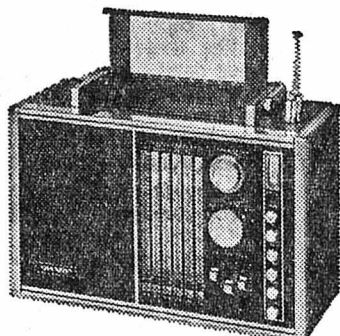
FV 1800 Radio spéciale pour ondes courtes, 11-120 m, OUC/S x OC/OM/OL, 17 transistors, sortie de 3, 5 Watt pile/secteur, 350 x 238 x 140 mm, 6,5 kg. Fr. 495.—
