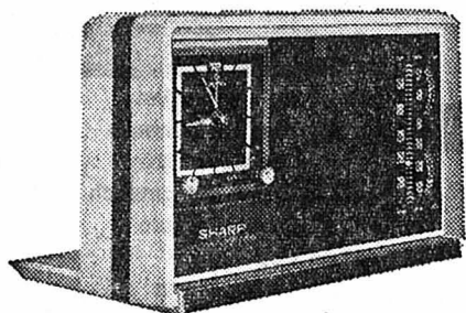
BXC 12 L Radio-réveil, OM/OL, 183 x 101 x 49 mm, 650 g Fr. 115.—
