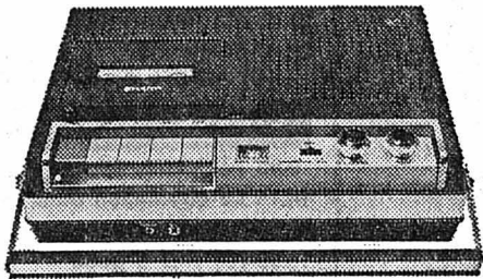
RD 403 Enregistreur à cassettes, piles et secteur, compteur, 284 x 205 x 69 mm, 2,1 kg Fr. 285.—
