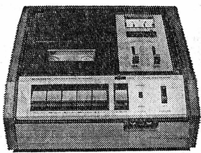
RD 423 Enregistreur à cassettes stéréo, «Tape Deck», compteur, prises DIN, 85 x 257 x 262 mm Fr. 465.—
