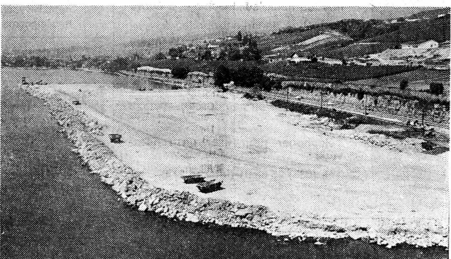
Le remblai s'avance, jour après jour, en direction du village d'Auvernier. (Avipress - J.-P. Baillod.)
