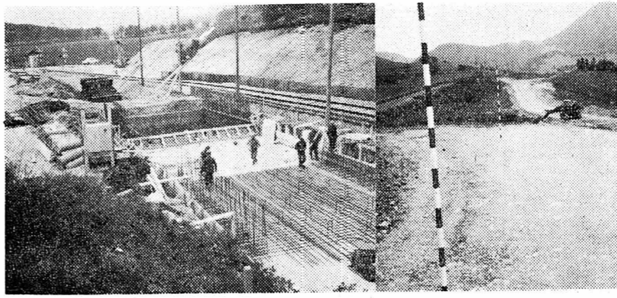
Les travaux de fondation d'un tunnel dans la région du Loclat (à gauche), et l'ébauche de la nouvelle route au nord du Loclat et du cimetière de Travers. (Avipress - FyJ)
