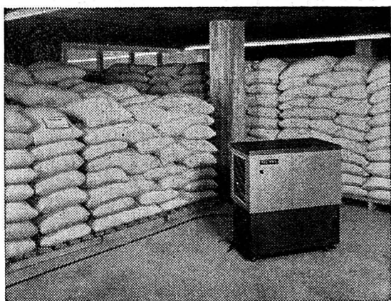
PRETEMA un déshumidificateur PR 200-HG dans un entrepôt de sucre
