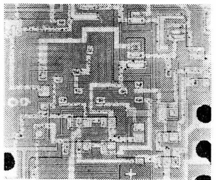
Le minuscule circuit imprimé ayant causé l'échec du lancement de « Mariner-8 » : l'une des connexions avait été rompue accidentellement. (Avispress - Cedos)
