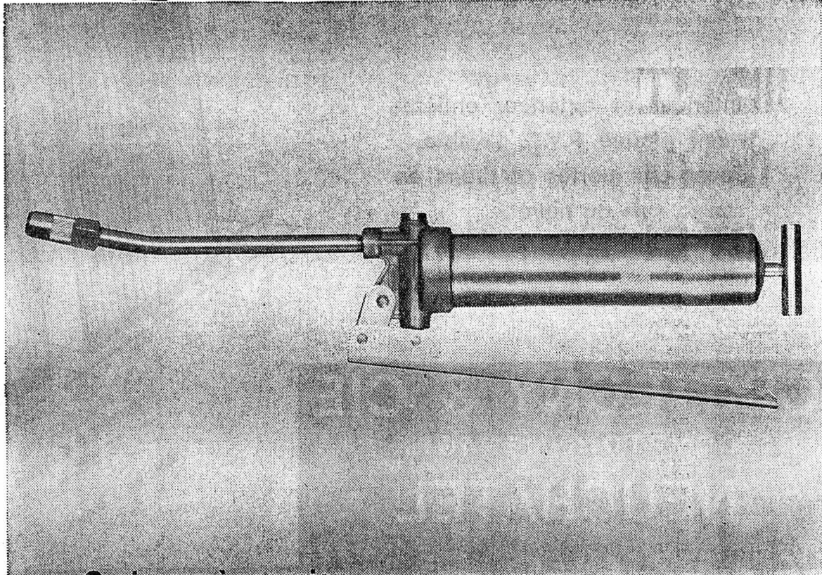
Graisseur à pression EMPEROR Exécution solide et pratique.
