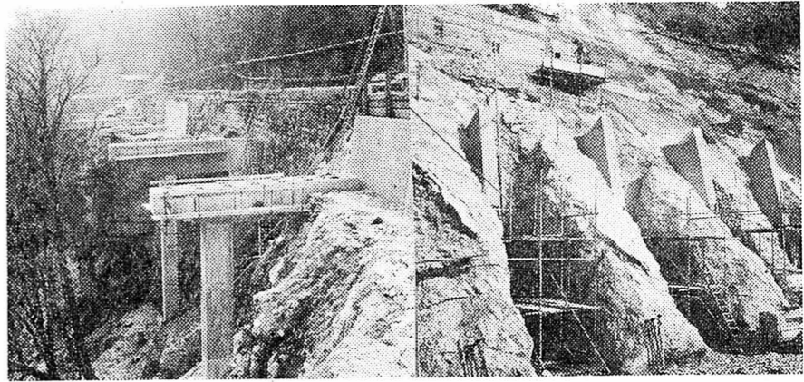
Sur les chantiers actuels: coulage de piliers de béton sur la route du Taubenloch, à gauche, et le long de la RN 5, à droite. (Avpress - Guggisberg)
