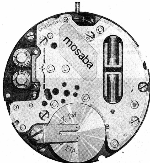
Mouvement électronique à résonateur de flexion de la 2 me génération
