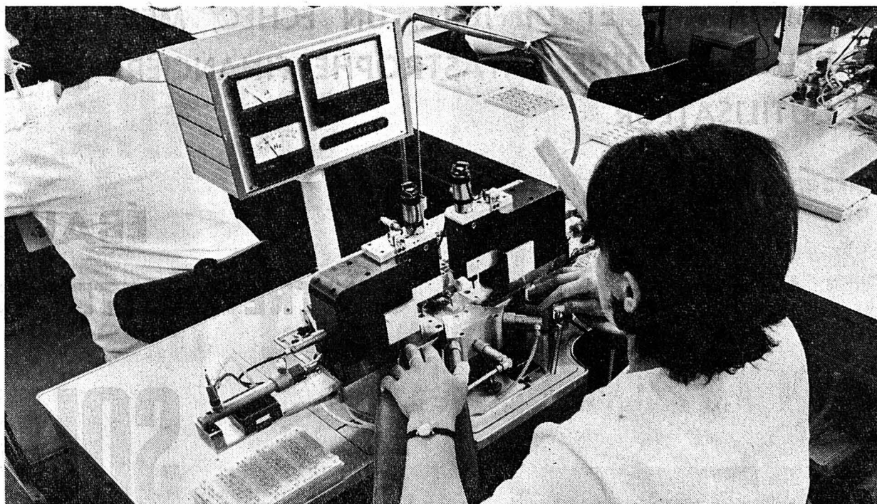
Symétrisation et mise à la fréquence des résonateurs
