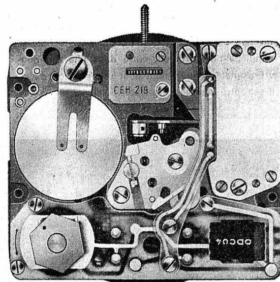
Mouvement électronique à quartz de la 3 me génération
