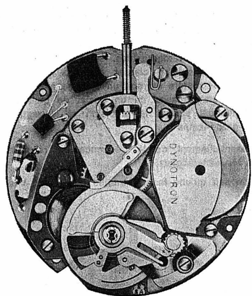
Mouvement électronique à balancier-spiral de la première génération
