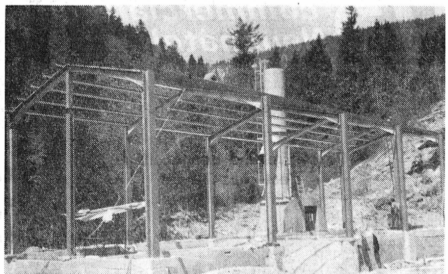
L'armature métallique de l'usine d'incinération des ordures et mise en place. A l'arrière-plan: la cheminée.
