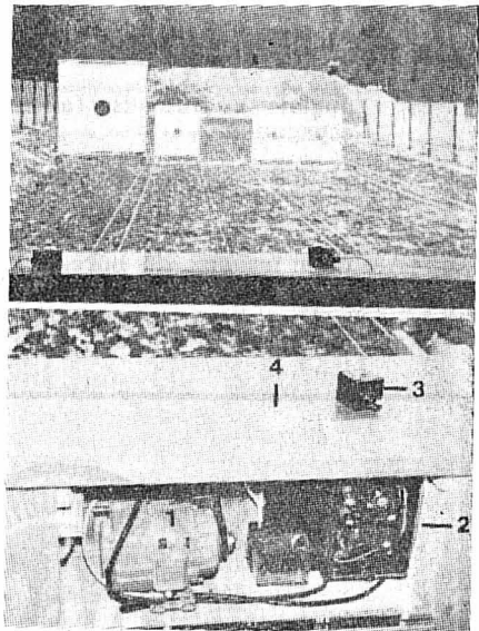
En haut : vue générale d'une ciblerie avec câbles et chariots. En bas : tableau de commande. 1. moteur électrique. 2. boîtier de commande électronique. 3. bouton de commande. 4. emplacement du compteur à monnaie (facultatif).
