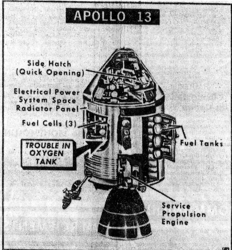
Ce dessin montre (flèche) l'endroit où la fuite d'oxygène s'est produite dans la cabine Apollo. A droite (fuel tanks) se trouvent les réservoirs de carburant. (Téléphoto AP)
