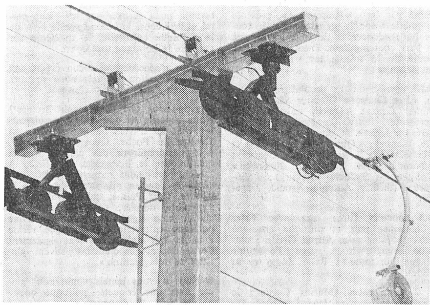
Rattrape-câble, arrêts automatiques, guides latéraux : tout a été prévu, mais pour un usage normal
