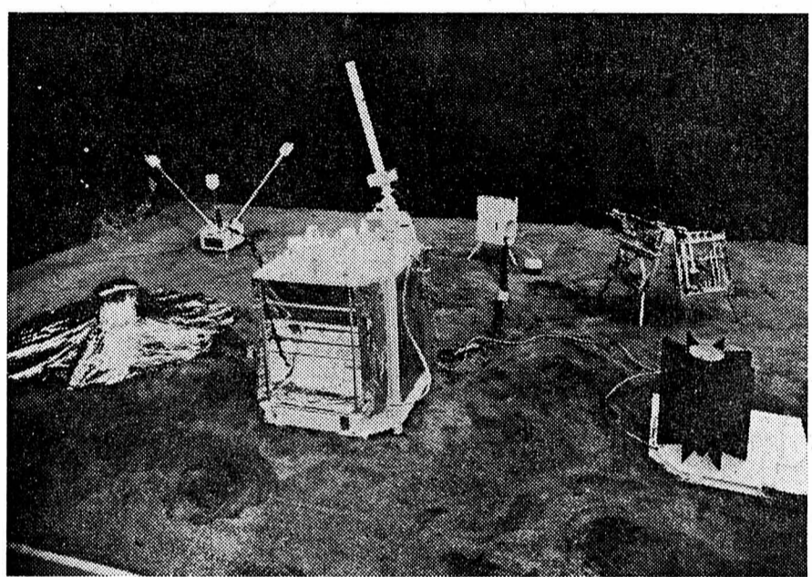
La disposition précise des différents appareils des astronautes d'Apollo 12 sur le sol lunaire. (De g. à dr.) L'appareil destiné aux expériences sismiques, le magnétomètre, le détecteur d'ions, les outils des astronautes rangés dans la mallette, le SNAP 27 et (premier plan, centre), la station centrale.
