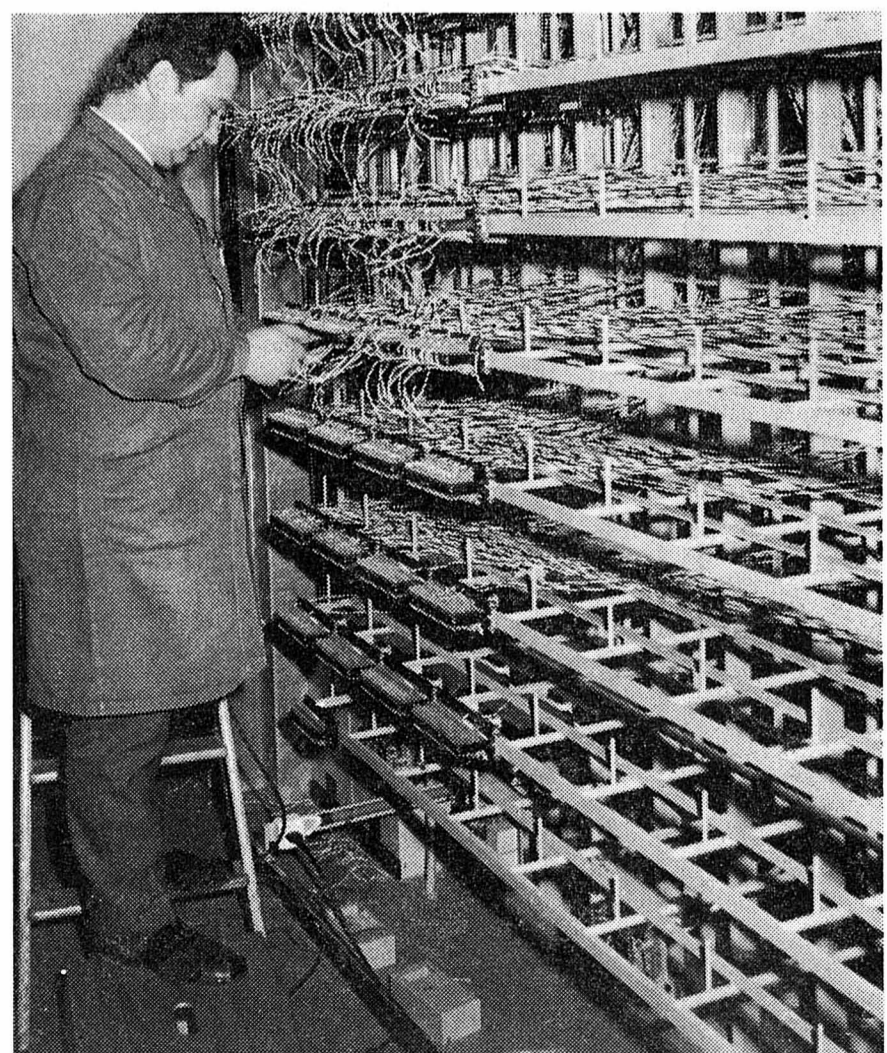
Chaque ligne d'abonné entrante est reliée par un double fil du distributeur principal aux équipements de central
