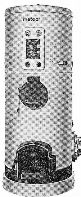
meteor II Chaudière combinée à double foyer, avec deux chambres de combustion indépendantes. Permet d'utiliser simultanément du mazout et des combustibles solides.
