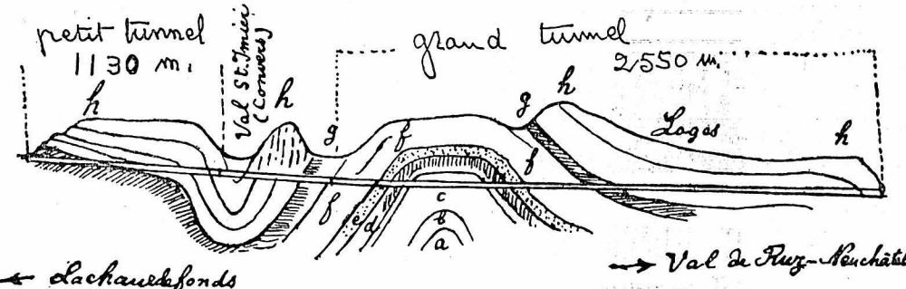
Coupe géologique des tunnels des Loges et du Mont-Sagne, d'après un croquis figurant dans une lettre de Gressly en 1855. (Extrait des « Lettres d'Amand Gressly, le géologue jurassien », éditées par le Dr Louis Rollier, Montier, 1911.)
