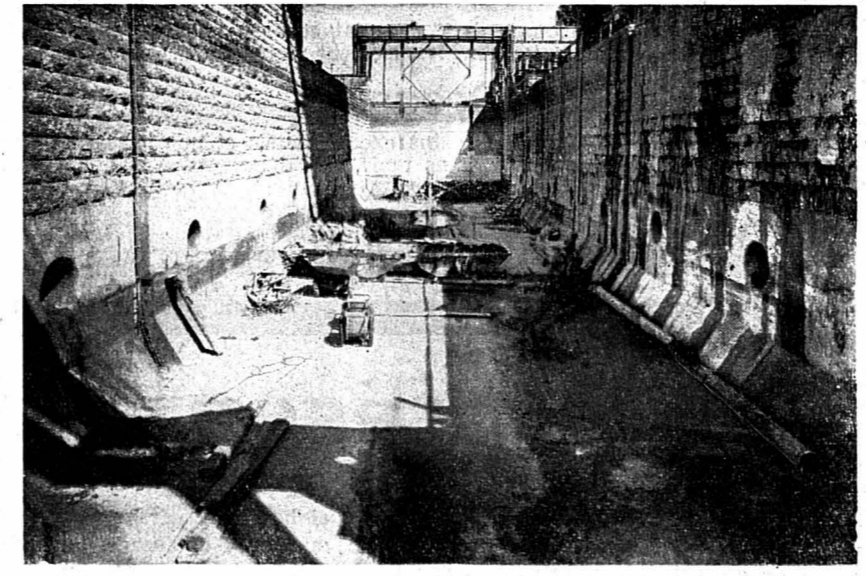
En vue de la II e correction des eaux du Jura, l'écluse de Nidau a été approfondie de 1 m 80. Les travaux ont été faits en avril et mai 1961.
