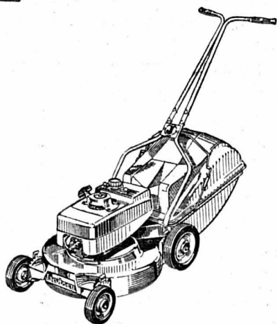
MODÈLE TURBI VAC démarrateur à ressort ramasse-herbe
