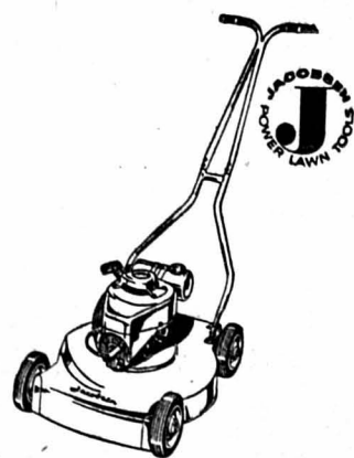
MODÈLE 63 C moteur silencieux
