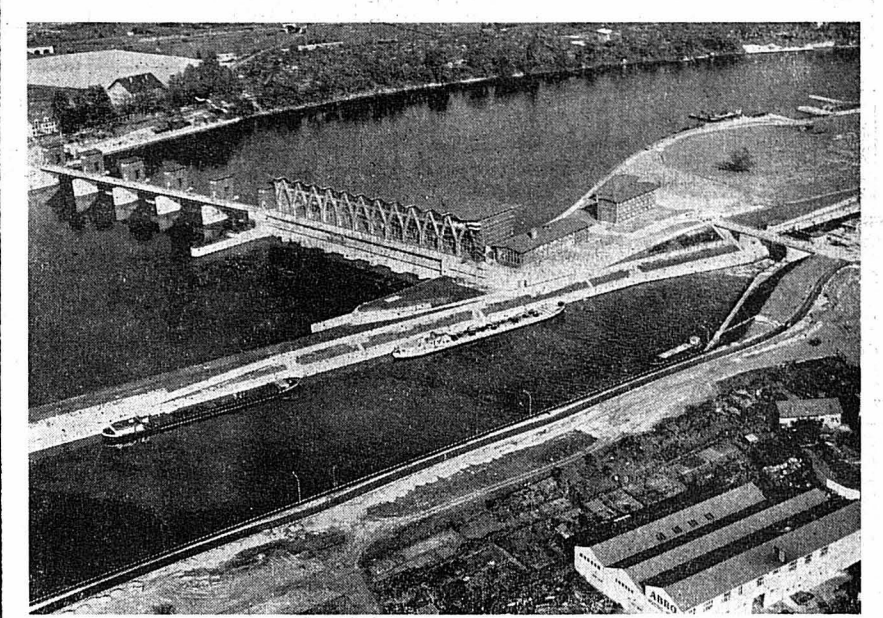
L'usine électrique de Birsfelden sur le Rhin, près de Bâle, dont la construction a duré cinq ans, a été mise en exploitation. Au premier plan : l'écluse pour la navigation.
