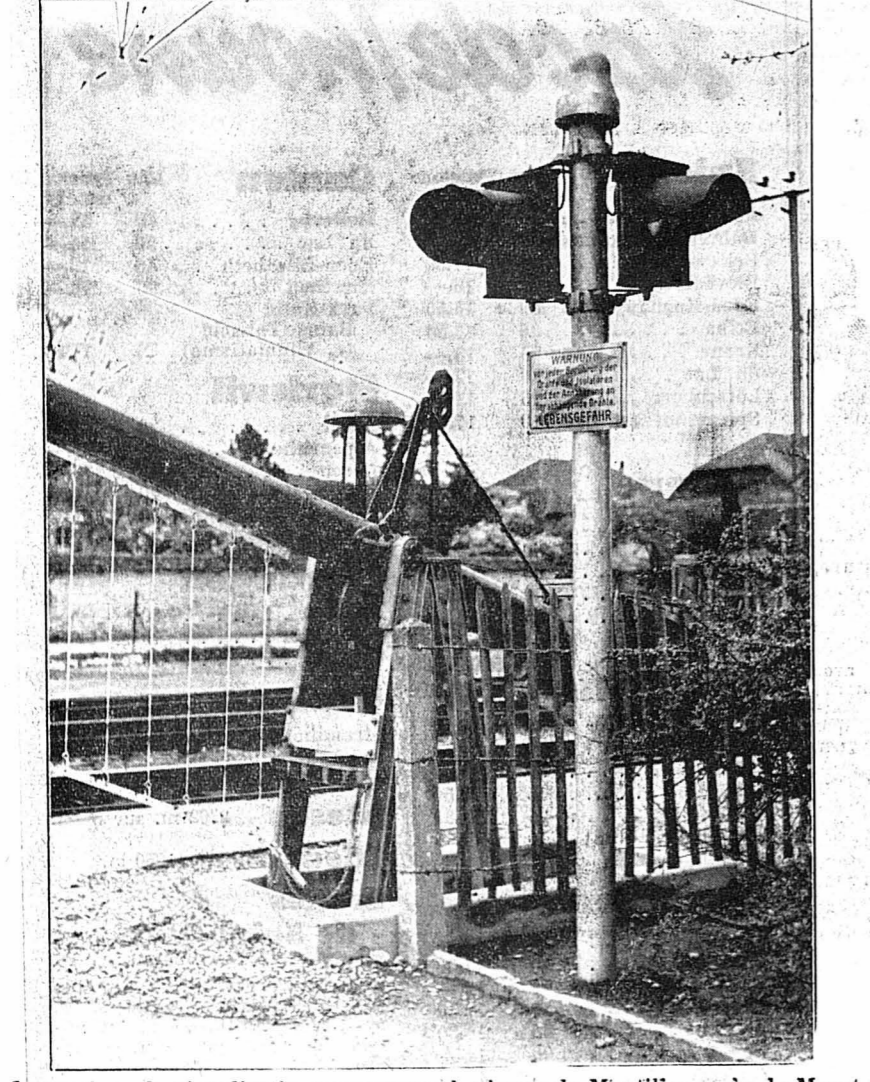
Le système de signalisation au passage à niveau de Montilier, près de Morat.
