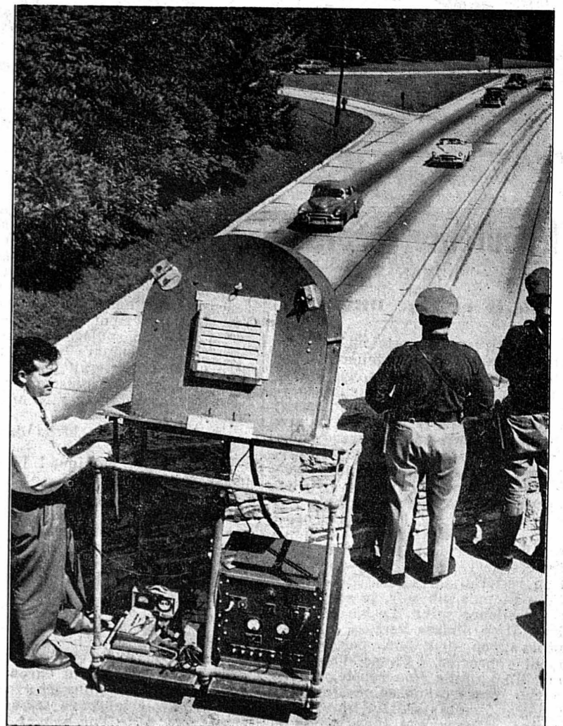
La police de l'Etat de New-York a mis en service un appareil de radar pour contrôler la vitesse des véhicules. Dès qu'un véhicule dépasse la vitesse prescrite, l'appareil se déclenche et une caméra filme l'automobiliste en contravention.
