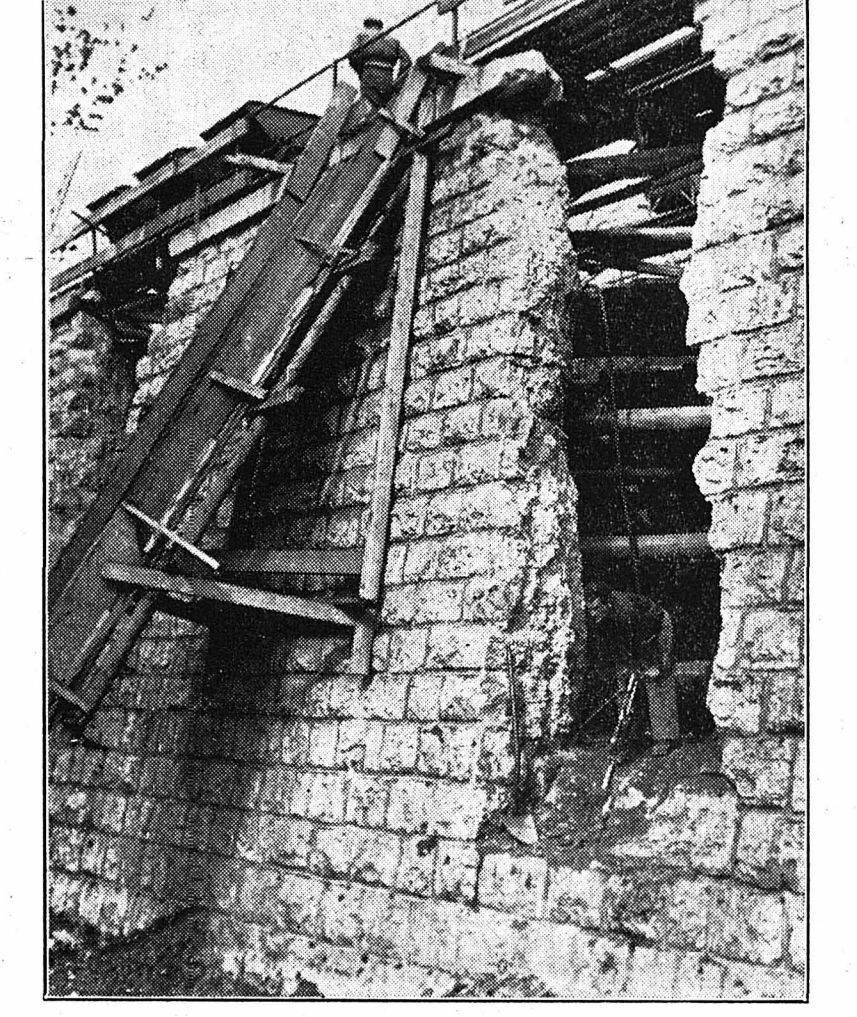
Voici l'ouverture centrale pratiquée dans le mur de soutènement de la ligne C. F. F. C'est là que seront posés six piliers sur lesquels on fixera la « palée intermédiaire ».
