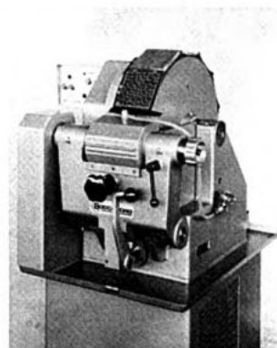
Machine à scier en carrés, cubes et listes Type ES 12
