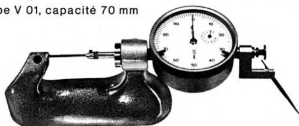
Type H no 02 capacité 0-20 mm, course 10 mm no 07 capacité 0-20 mm, course 10 mm no 08 capacité 0-30, course 30 mm
