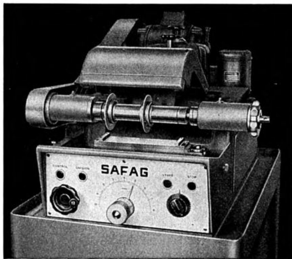
Type 32 1 à 8 scies pour le sciage des boules, demi-boules, barreaux, etc.
