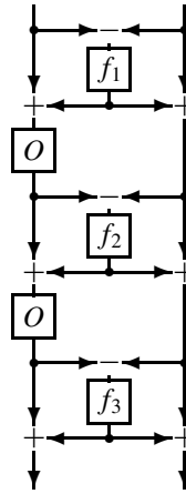
Fig. 7. Lai-Massey scheme.
