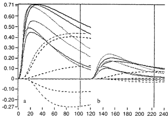
Bild 6. Geruchsprofile mit 12 Sensoren, aus frischem Holz der Fichte. X-Achse: Zeit; Y-Achse: Variation des Sensorwiderstands (k-Ohm). A: Splintholzprobe B: Kernholzprobe, aus dem Juvenilbereich (Zeitachse verschoben)
