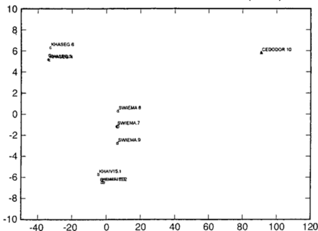
Bild 4. 2-dimensionale Unterscheidung von afrikanischen und amerikanischen Vertretern der Meliaceen. Khaseg: Khaya senegalensis , Gambia-Mahagoni; Khaiv: Khaya ivorensis , Afrik. Mahagoni; Swiema: Swietenia macrophylla , Amerik. Mahagoni; Cedodor: Cedrela odorata , Cedro
