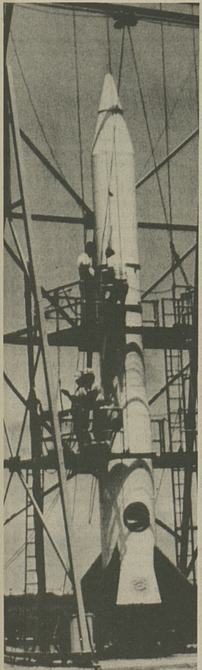
Le lanceur «Conestoga-1» sur son pas de tir à Matagorda Island (Texas). (Keystone)
