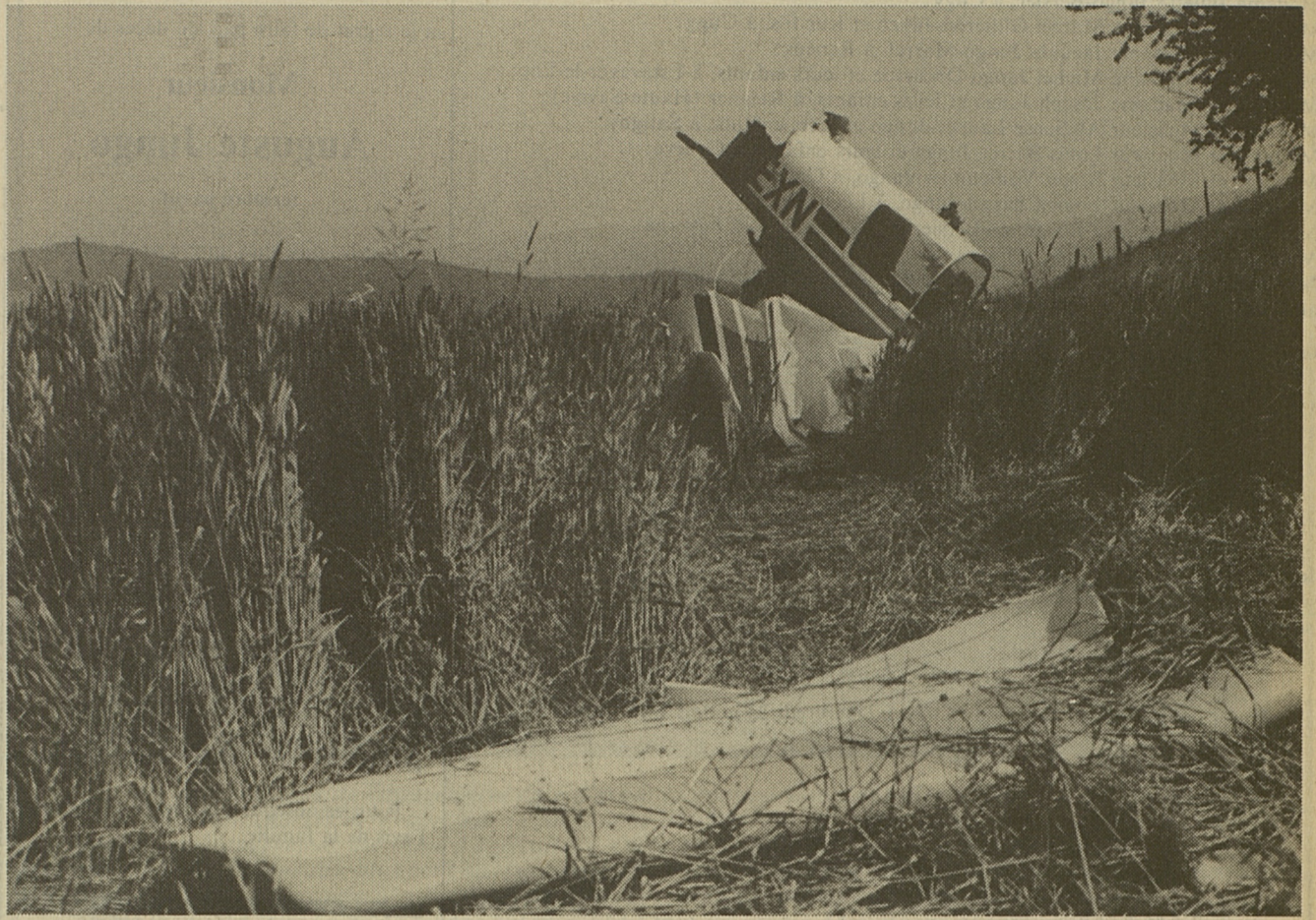
Au premier plan, l'aile brisée; au fond, ce qu'il reste du Robin immatriculé HB-EXN
