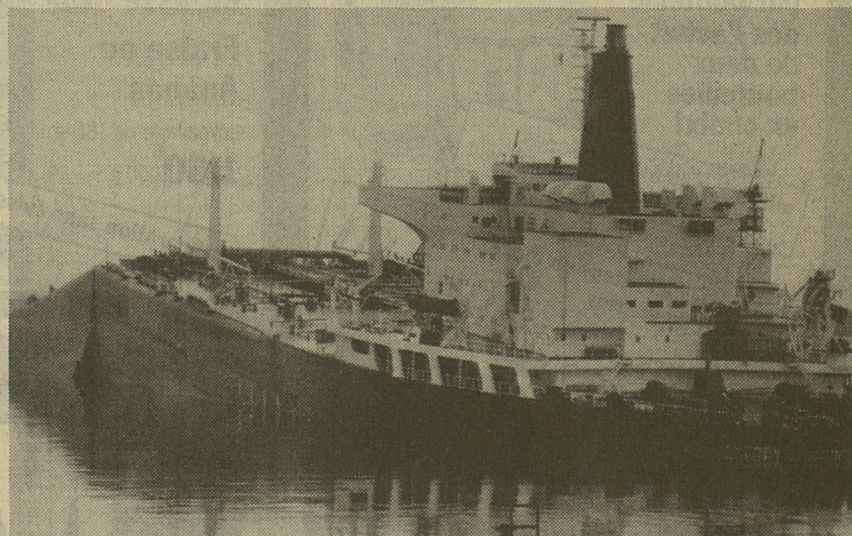
Le bateau libérien «Energy Concentration», qui s'est brisé en deux dans le port de Rotterdam, à la suite d'une fausse manœuvre dans le déchargement de ses 220 000 tonnes de pétrole. (Keystone)
